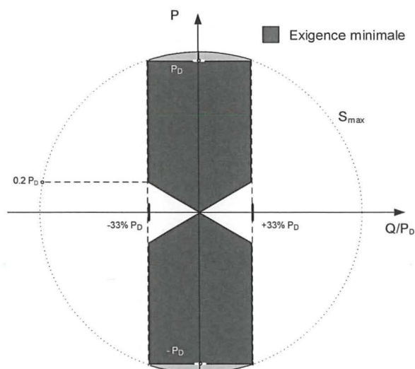
Capacité réactive pour installation de stockage d'énergie non-synchrone Type B.
