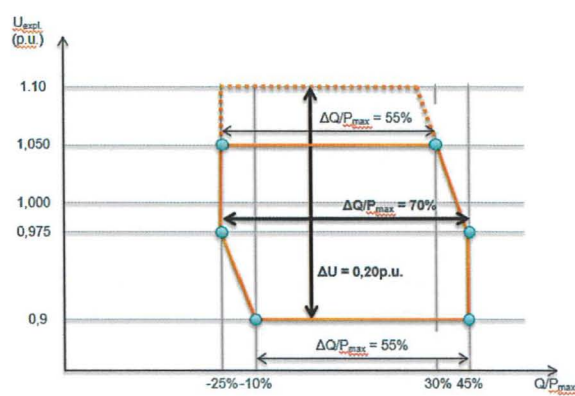
U-Q/P_D -profiel voor SPM van het type C en D: vereisten met betrekking tot het reactief vermogen voor verschillende spanningsniveaus (gestippeld voor nominale spanningen boven 300 kV).
