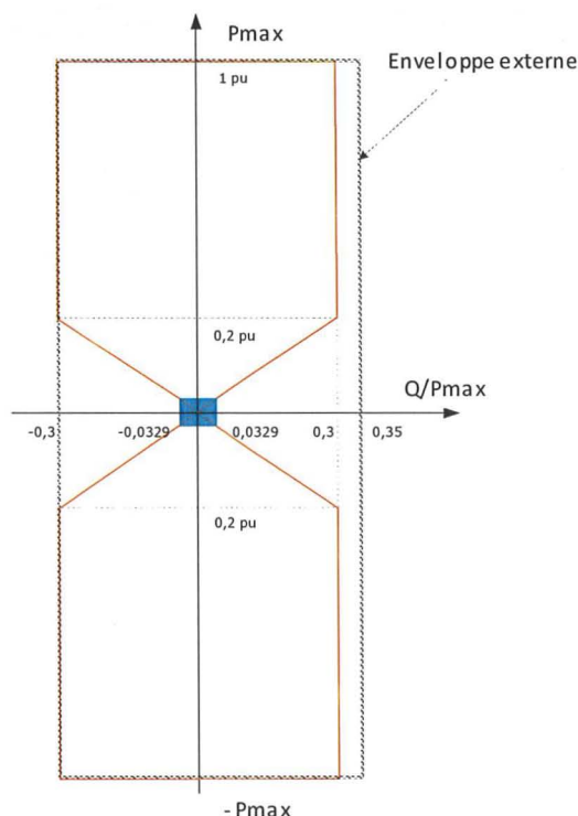
Capacité réactive pour installation de stockage d'énergie non-synchrone type C et D.
