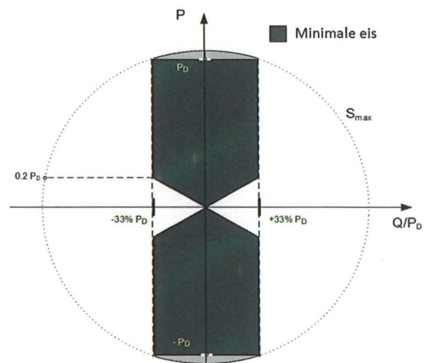
Reactieve capabiliteit voor asynchrone energieopslagfaciliteit type B.
