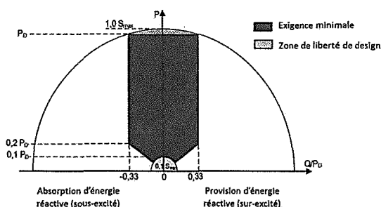
Courbe de capacité pour les SPGM de type B.
