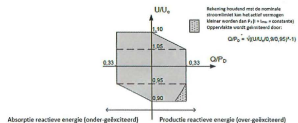
U-Q/P D -profiel voor SPM van het type B: vereisten met betrekking tot het reactief vermogen voor verschillende spanningsniveaus.
