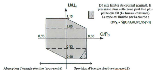
Profil U-Q/P D pour SPM types B : exigences relatives à la puissance réactive pour différents niveaux de tension ;
