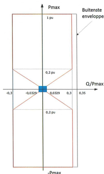
Reactieve capaciteit voor asynchrone energieopslagfaciliteit type C en D.
