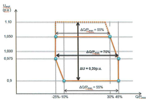
Profil U-Q/P_D pour SPM types C et D : exigences relatives à la puissance réactive pour les niveaux de tension (pointillé pour les tensions nominales au-dessus de 300 kV).
