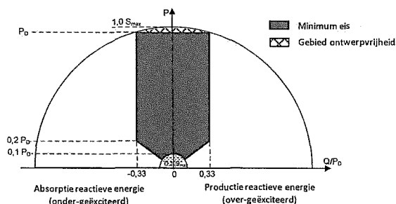
Capaciteitscurve voor SPGM type B.
