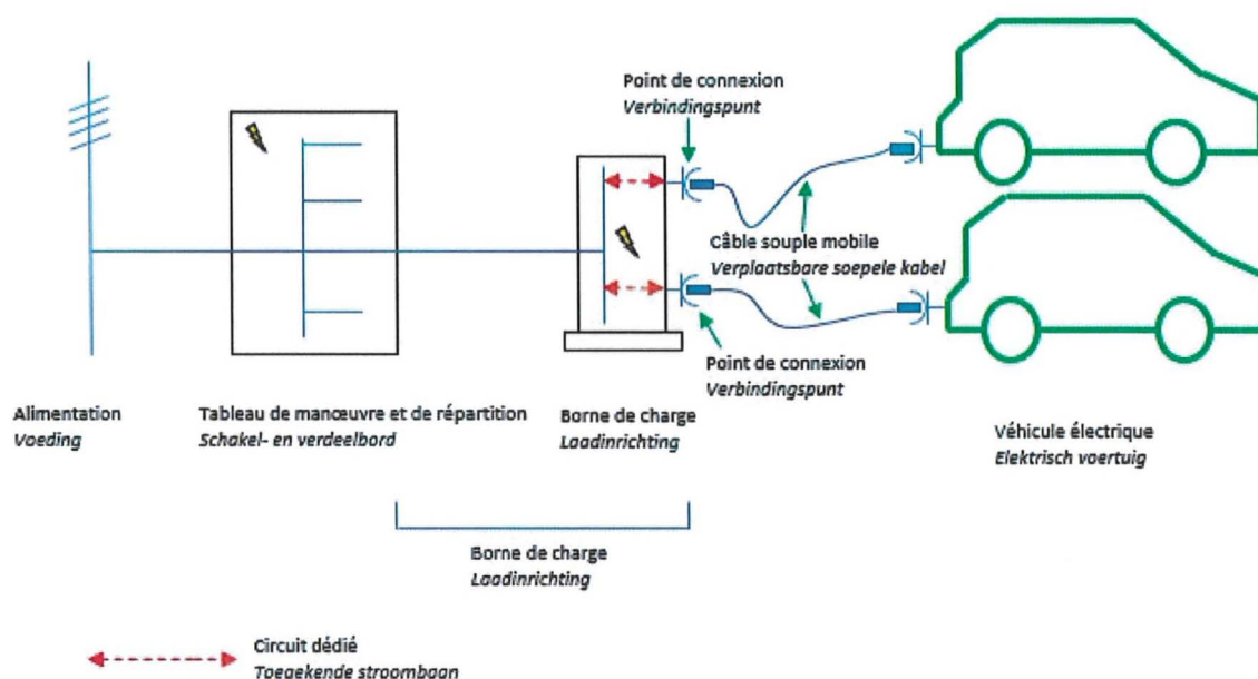
Figure 7.20. Borne de charge avec deux points de connexion « socles de prise de courant sur borne de charge » faisant partie de la borne de charge (dispositifs de protection contre les surintensités des circuits dédiés intégrés dans la borne de charge)
