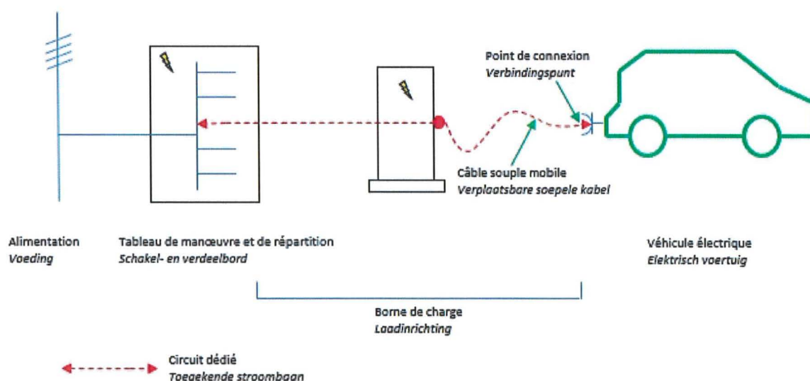
Figure 7.17. Borne de charge avec un point de connexion « prise mobile de véhicule » faisant partie de la borne de charge (dispositif de protection contre les surintensités du circuit dédié intégré dans le tableau de manœuvre et de répartition) Figuur 7.17. Laadinrichting met één verbindingpunt "voertuigconnector" dat deel uitmaakt van de laadinrichting (overstroombeschermingsinrichting van de toegekende stroombaan geïntegreerd in het schakel- en verdeelbord)
