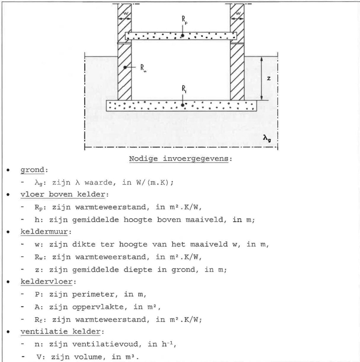
Figuur [48]: Schildelen van een kelder
