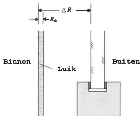
Figuur [18]: Venster met gesloten luik
