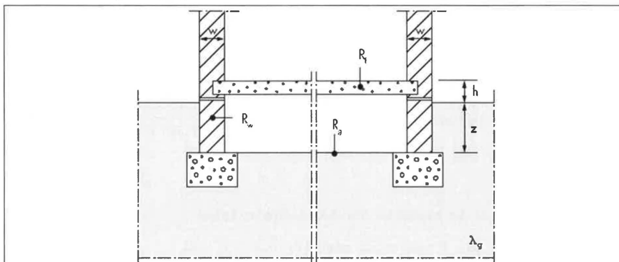
Figure [47] : Planchers au-dessus d'un vide sanitaire
