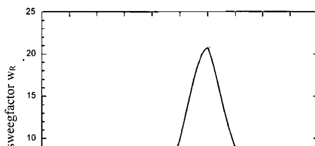
Figuur X : de stralingsweegfactor w_R voor neutronen versus neutronenergie.
