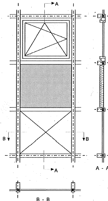
Figuur [20]: Module van een lichte gevel (gordijngevel)
