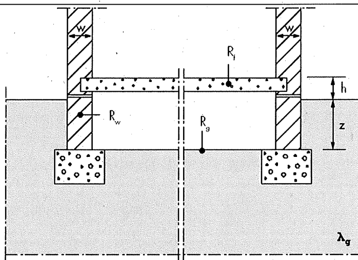
Figure [47] : Planchers au-dessus d'un vide sanitaire
