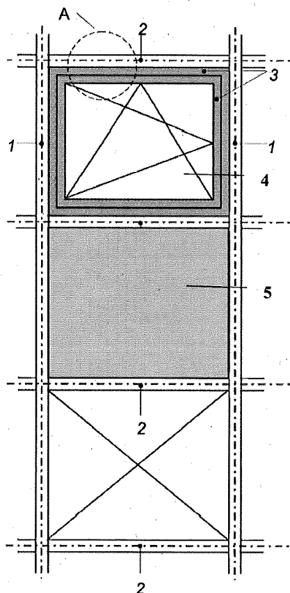
Figuur [21]: Samenstellende delen van een gordijngewel
