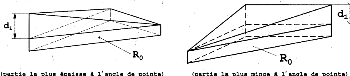
Figure [8] : Éléments de construction avec base triangulaire, composés d'une partie inclinée et d'une partie plane (restante)
