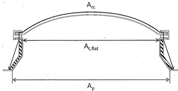
Figuur [51]: Oppervlaktes van een lichtkoepel met opstand
