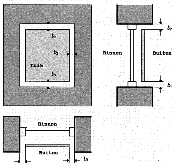
Figuur [19]: Karakteristieken van luchtspleten rond gesloten luiken
