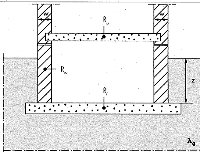
Figuur [48]: Schildelen van een kelder
